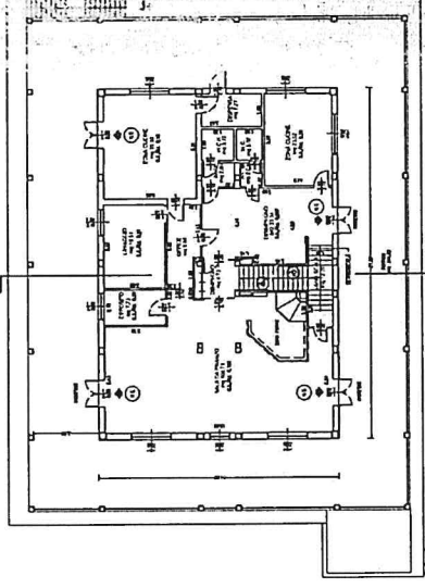
Pianta Piano Terra Scala 1:100
